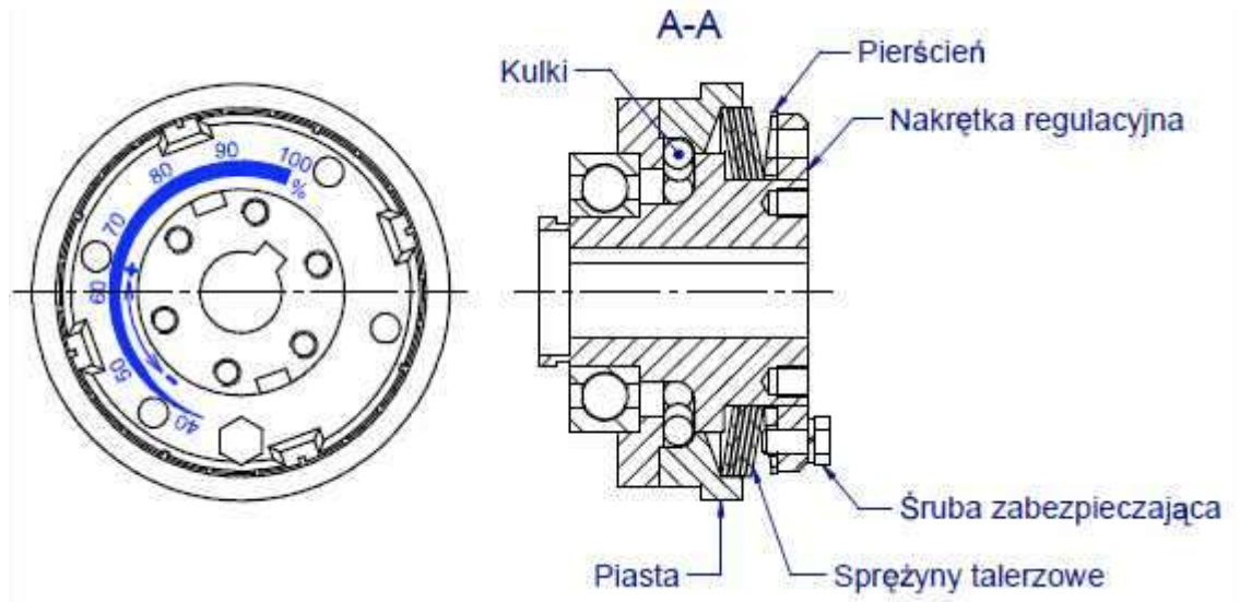
Rys. 45. Sprzęgło EAS-comp.01/490.720.0
